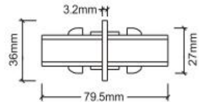
3線A 迷你型直綫接駁器 Straight connector MINI
