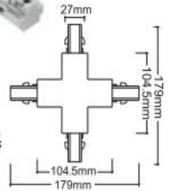
3線A 四向接駁器 X-Connector
