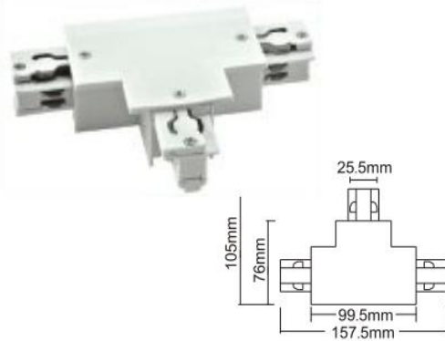
H-03 三向接駁器(左) T-Connector-L
