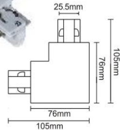
H-03 90° 接駁器(左) L-Connector-L
