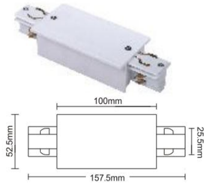
H-03 直線接駁器 Straight connector
