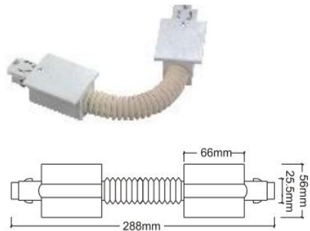
H-03 多角度接駁器(軟接) Flexible Connector
